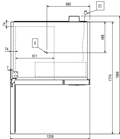
Boven aanzicht
